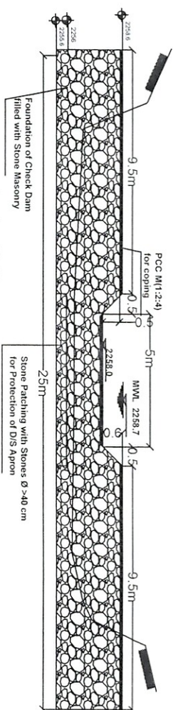
Section A3-A3 Scale 1:50
